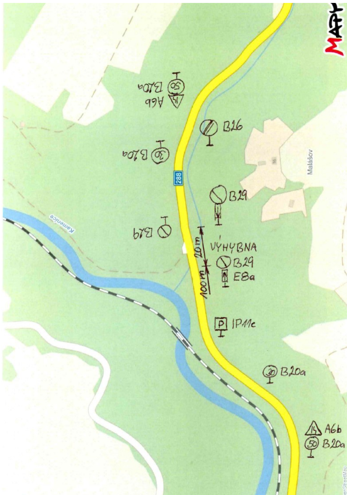
Příloha: Schéma umístění DZ ke stanovení čj. OD/1718/16 ze dne 15.04.2016.
